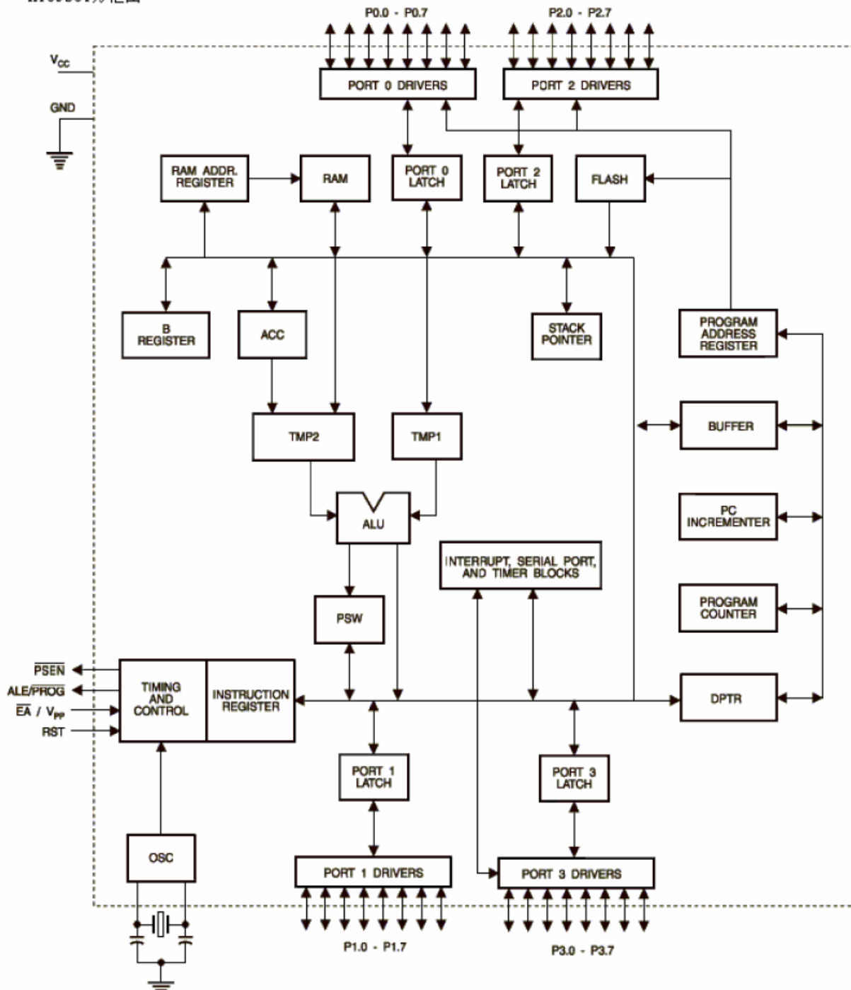
AT89S51方框图
